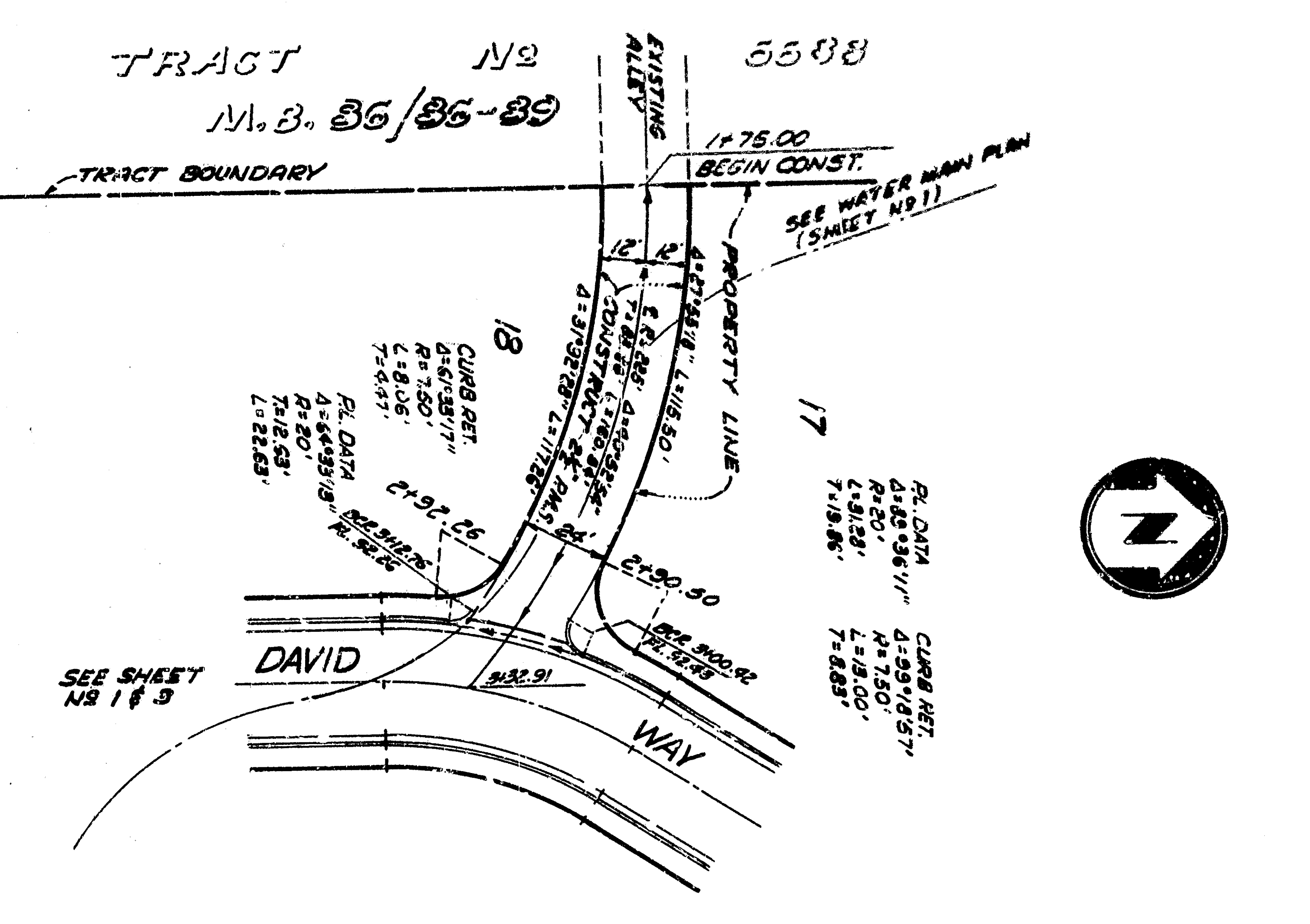
PLAN - ALLEY SCALE: 1" = 40'
